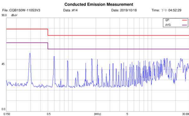
CQB150W-110S3V3-CMFC(D) Positive
