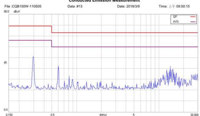
CQB150W-110S05-CMFC(D) Negative
