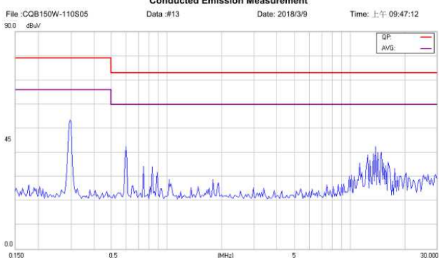
CQB150W-110S05-CMFC(D) Positive
