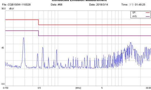
CQB150W-110S28-CMFC(D) Positive
