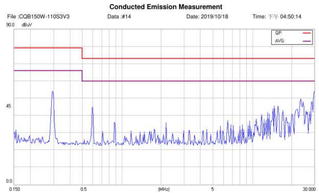
CQB150W-110S3V3-CMFC(D) Negative
