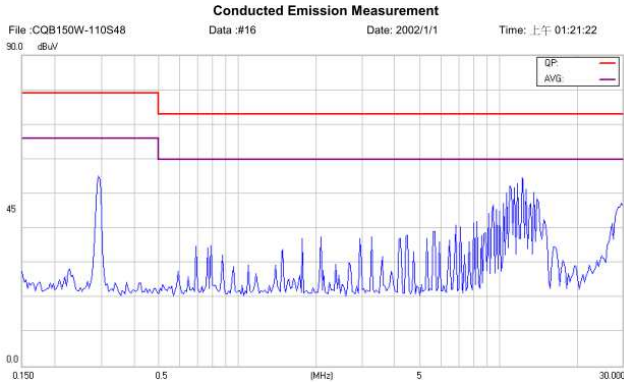
CQB150W-110S48-CMFC(D) Positive
