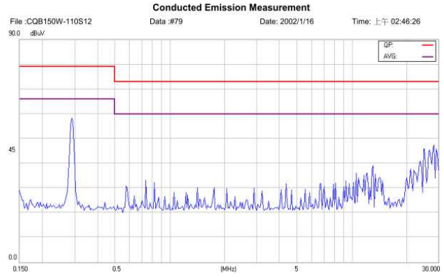
CQB150W-110S12-CMFC(D) Negative
