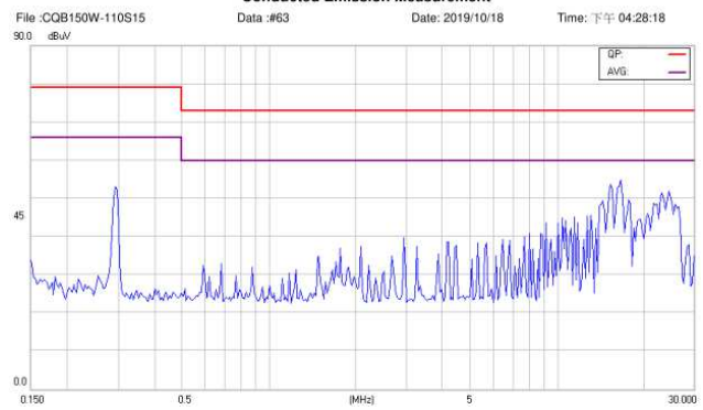
CQB150W-110S15-CMFC(D) Negative
