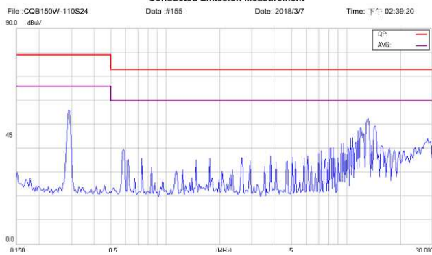
CQB150W-110S24-CMFC(D) Positive
