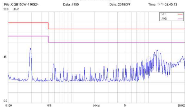
CQB150W-110S24-CMFC(D) Negative
