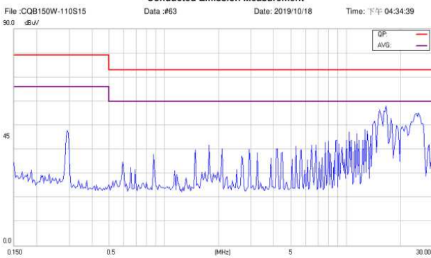
CQB150W-110S15-CMFC(D) Positive
