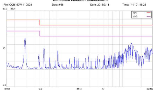
CQB150W-110S28-CMFC(D) Negative
