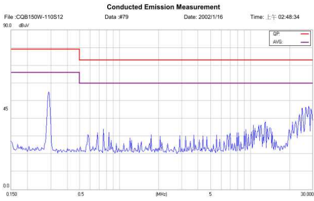
CQB150W-110S12-CMFC(D) Positive
