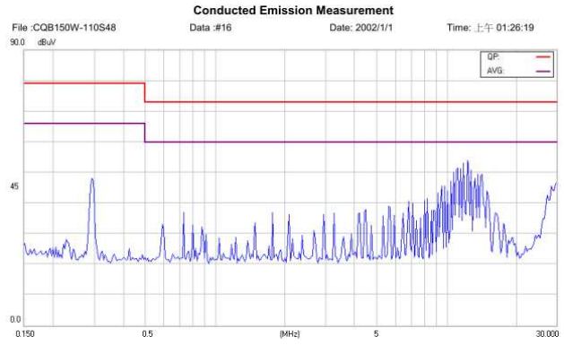
CQB150W-110S48-CMFC(D) Negative
