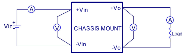
CHB300-300SXX-CMFC(D) Series Test Setup
